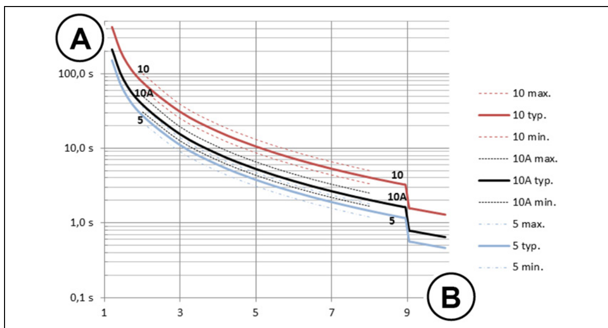
Рис. 1: Характеристики классов отключения
