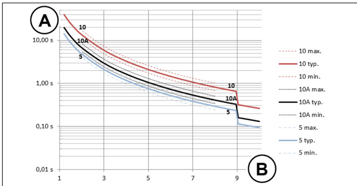
Рис. 2: Время отключения в разогретом рабочем состоянии (если до этого: I = \text{продолжит. } I_{\text{ном}} )
