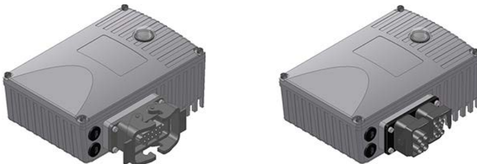
Rysunek 12: Przykłady urządzeń ze złączami wtykowymi dla przyłączy zasilania
