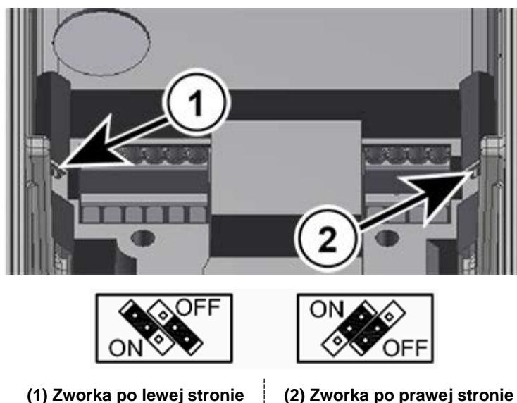
Rysunek 7: Zworki sieci zasilającej
