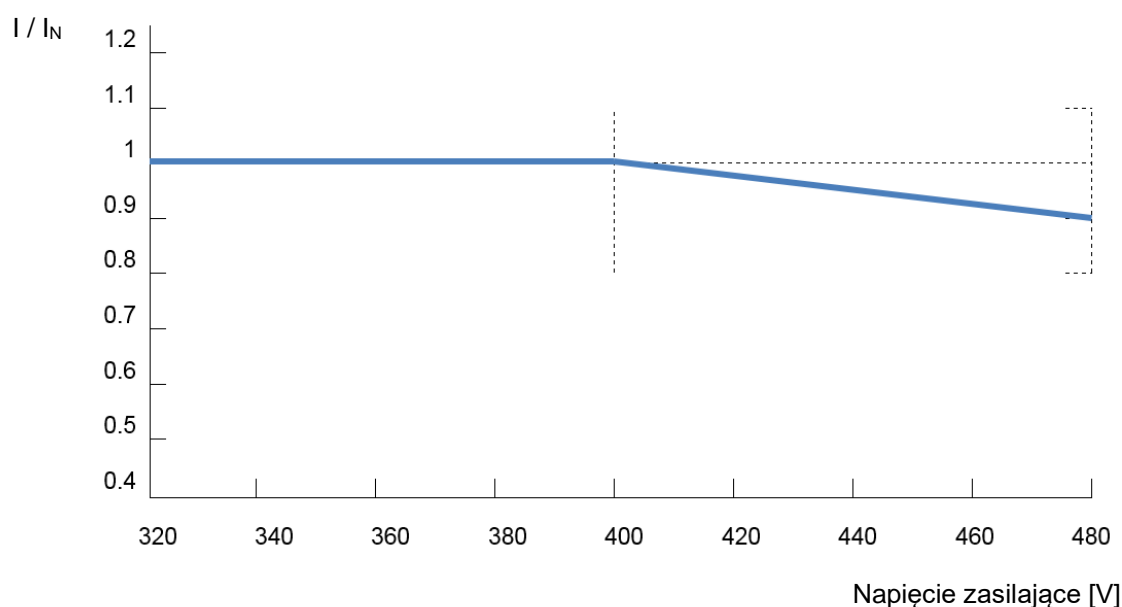
Rysunek 19: Prąd wyjściowy w zależności od napięcia zasilającego
