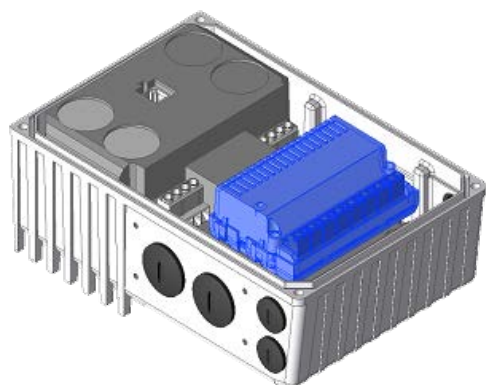
Rysunek 1: Urządzenie z wbudowanym SK CU4-...
