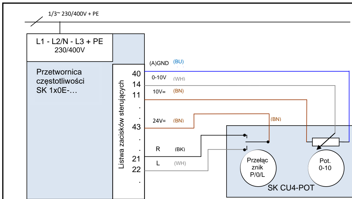
Rysunek 13: Schemat podłączeń SK CU4-POT, przykład SK 1x0E
