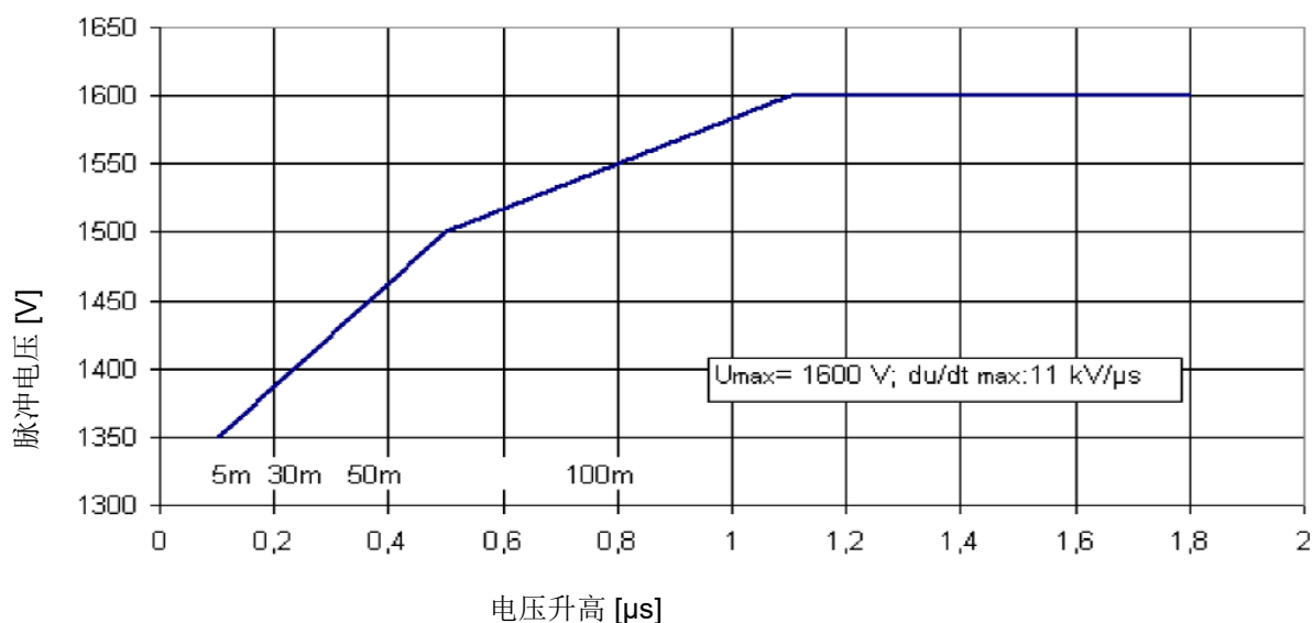
允许的脉冲电压取决于电压上升时间
